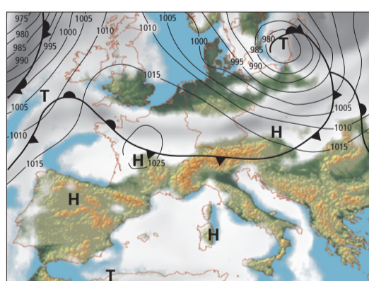
Bewölkung und Luftdruck heute H Hochdruckzentrum T Tiefdruckzentrum
